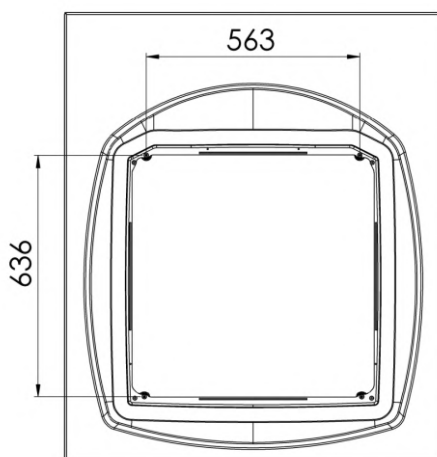
Kuva 1. Kiinnityspisteiden mitat
