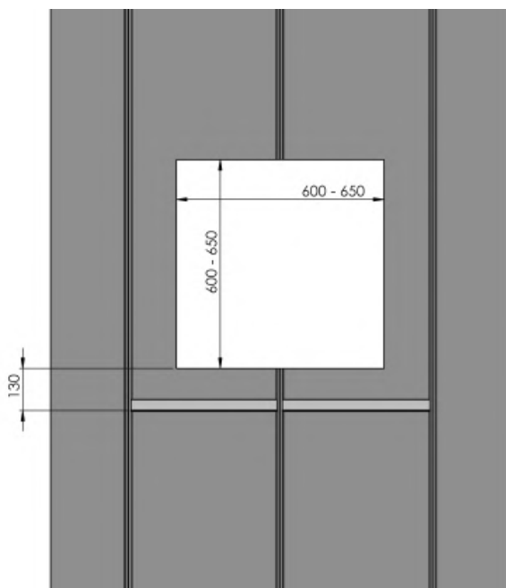
Kuva 5. L-Kulmien paikoitus pystysaumakatteeseen
