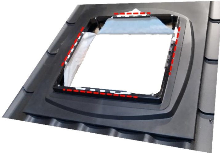
Kuva 7. Leikattu aluskate kiinnitettynä
